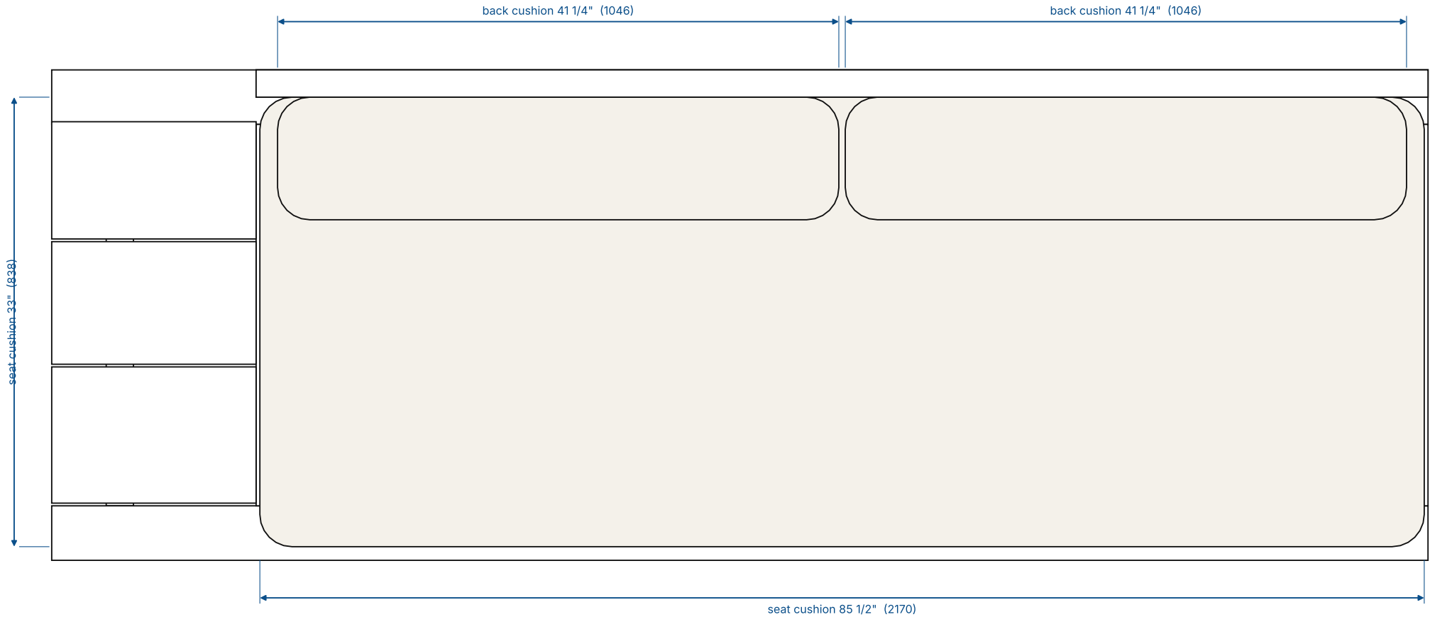
PLAN 1:10
